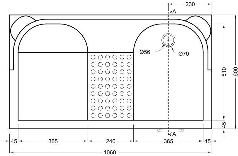
PIANTA
