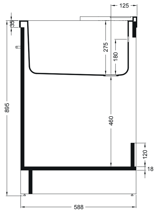
SEZIONE A-A
