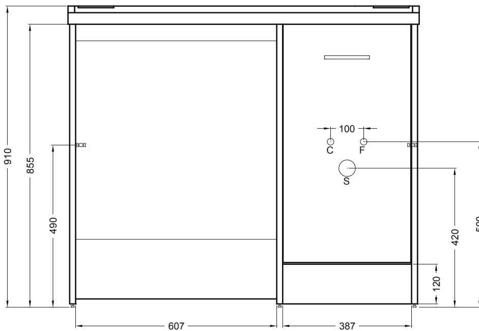
VISTA FRONTALE
