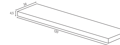
GRADINO PLUS ANGOLARE DX* 34x120x4,5 cm Rect - 13 3/8 "x48"x1 3/4 " LUX ± 9,5 mm
