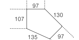
elemento pentaforme da 188 dx L. 188 P. 159 H. 44
