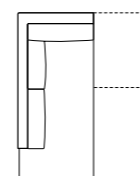
terminale ang. da 101x220 dx/sx L. 101 P. 220 H. 87
