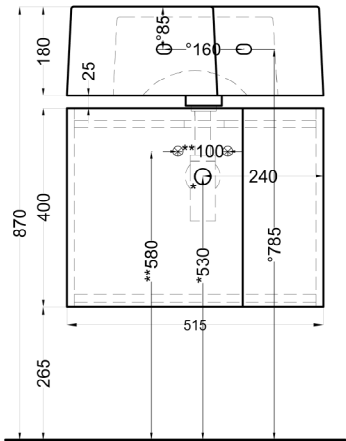
PROSPETTO FRONTALE
