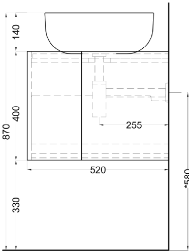
PROSPETTO LATERALE
