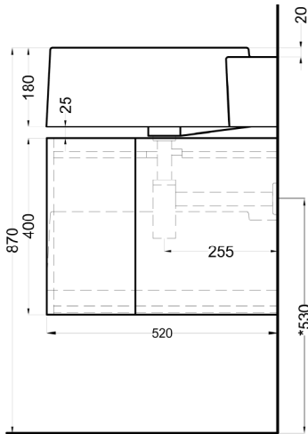
PROSPETTO LATERALE
