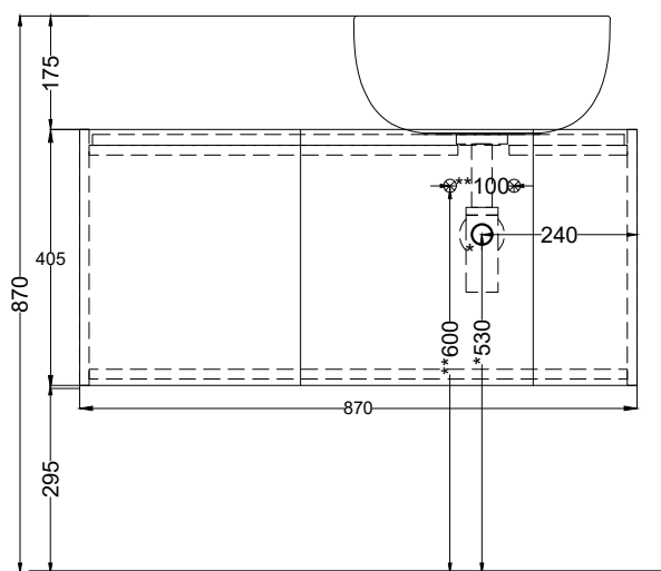
PROSPETTO FRONTALE
