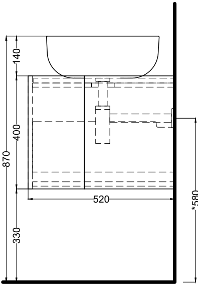
PROSPETTO LATERALE
