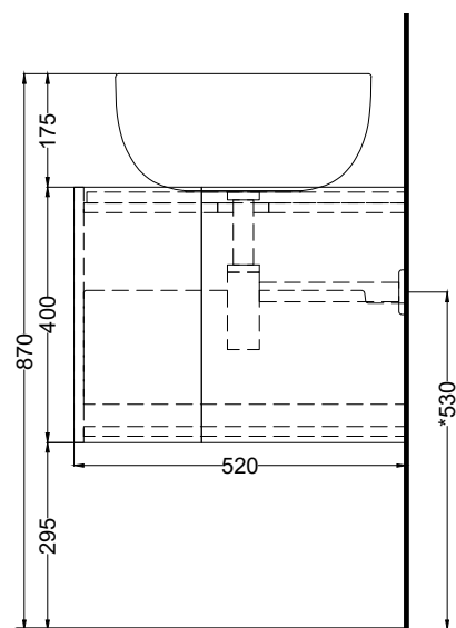
PROSPETTO LATERALE
