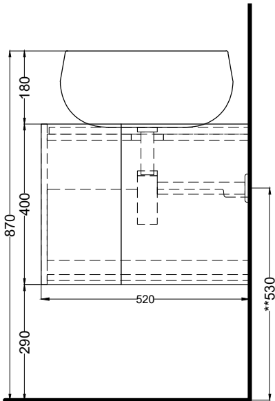
PROSPETTO LATERALE
