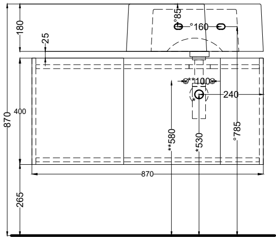
PROSPETTO FRONTALE
