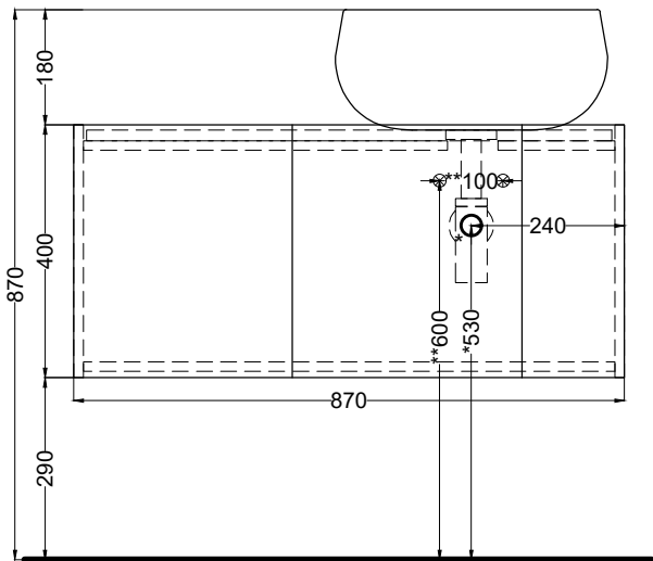
PROSPETTO FRONTALE
