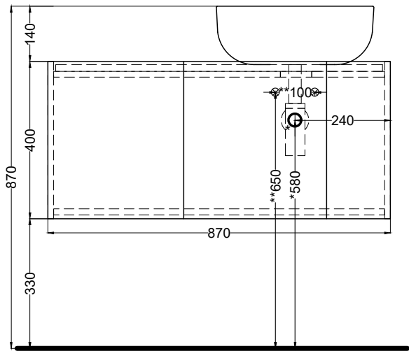
PROSPETTO FRONTALE
